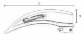
Macintosh Fiber Optic (F.O.) Laryngoscope Blades. (Fix Tube)
